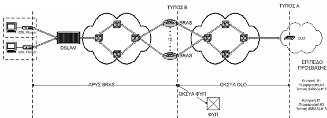
Σχήμα 1 Τύποι πρόσβασης
